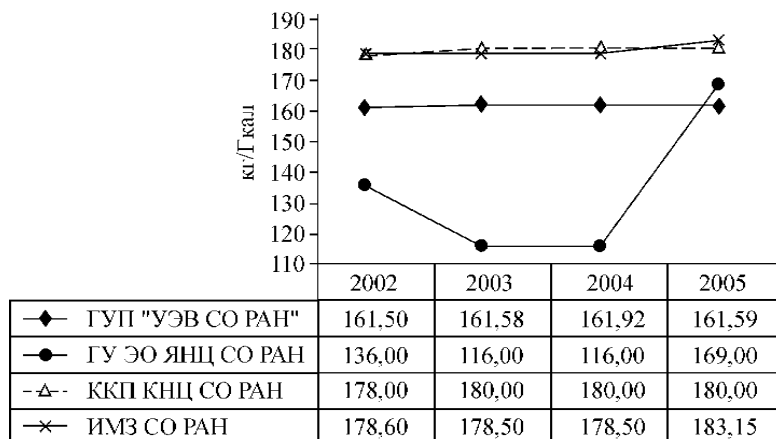
Рис. 4. Динамика удельного расхода условного топлива на 1 Гкал за 2002–2005 гг.
