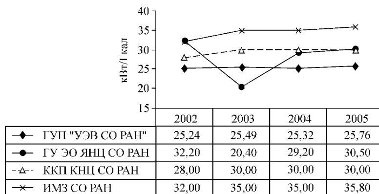
Рис. 5. Динамика удельного расхода электроэнергии на 1 Гкал за 2002–2005 гг.
